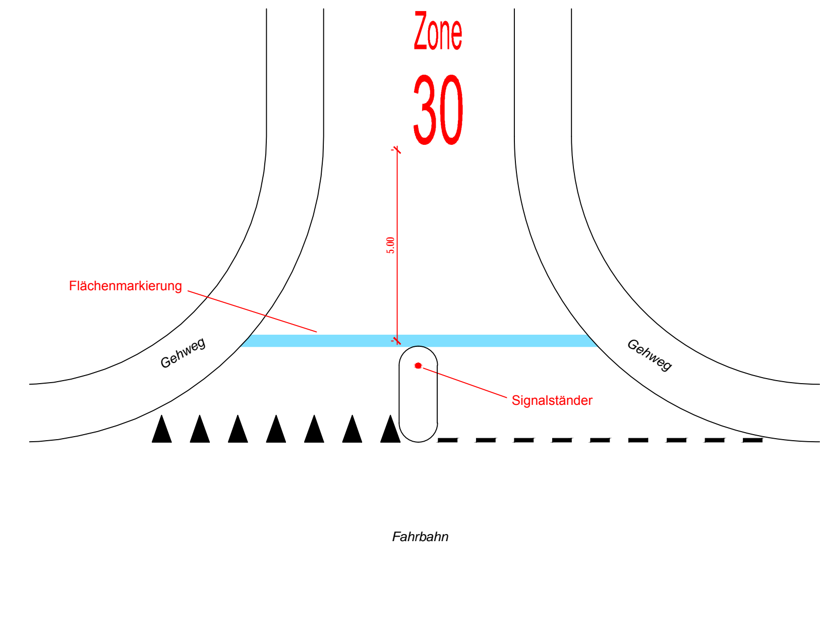
Detail Eingangstor Masstab 1:100
